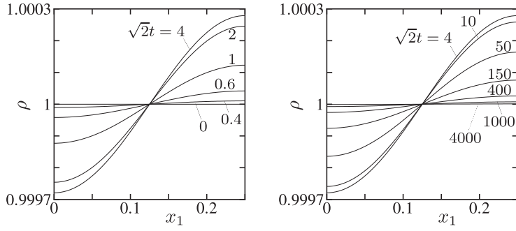
(d) \rho ( \sqrt{2}t \leq 4000 )
